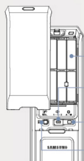
12 電池蓋 Battery Cover 13 關門鍵 Close Button 14 鹼性電池 x 8 AA (LR6) alkaline batteries 15 音量控制鍵 Sound Control Switch 16 自動/手動鎖定鍵 Auto/Manual Locking Switch 17 登記按鈕 Registration Button
