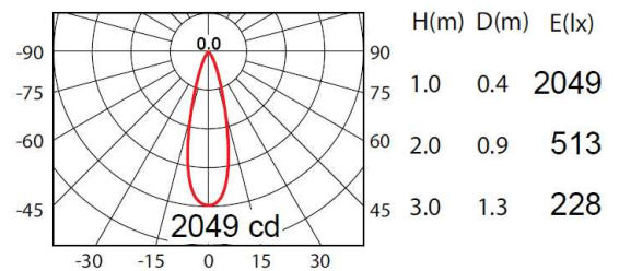
CoB 700lm 350mA WW 24°
