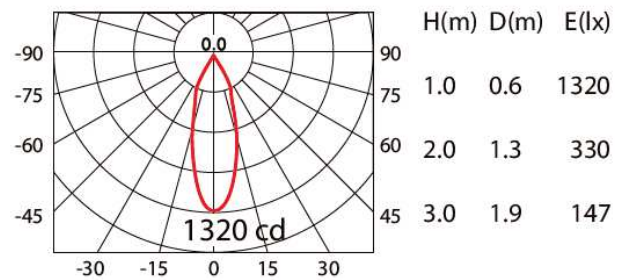
CoB 700lm 350mA WW 36°
